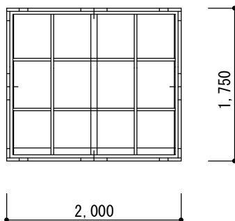
底側 平面図
